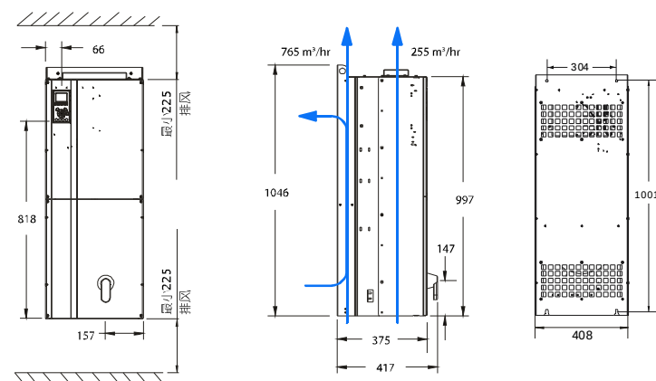
D3机箱 IP00
