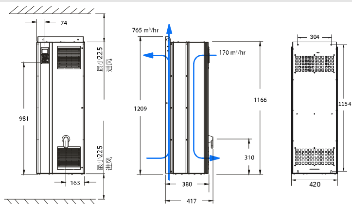
D1机箱 IP21/54
