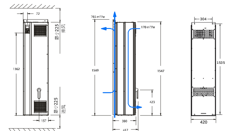
D2机箱 IP21/54
